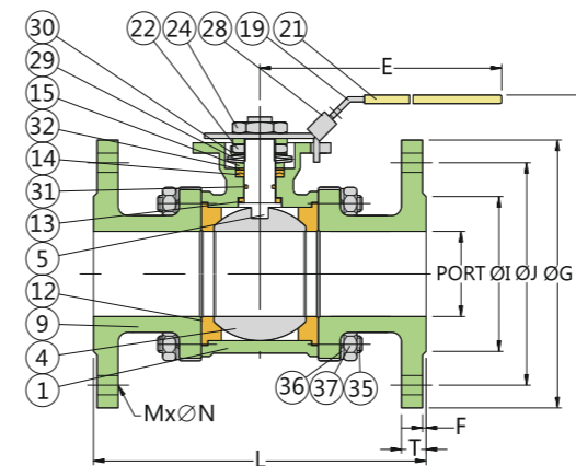
PN16 DIMENSIONS
